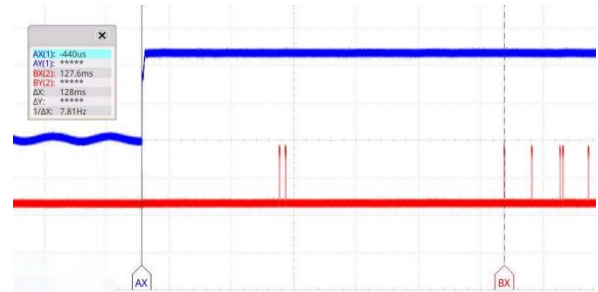
图 5-8. 样品 8 启动时间测试曲线
