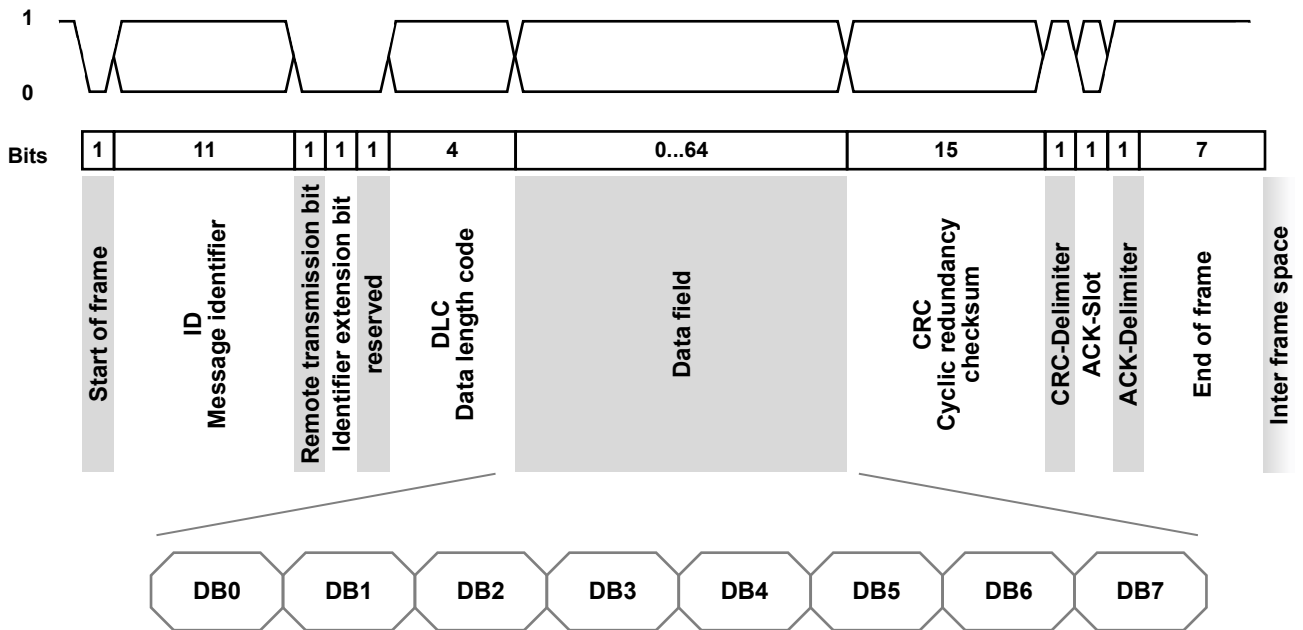
图 7-1. 标准帧
