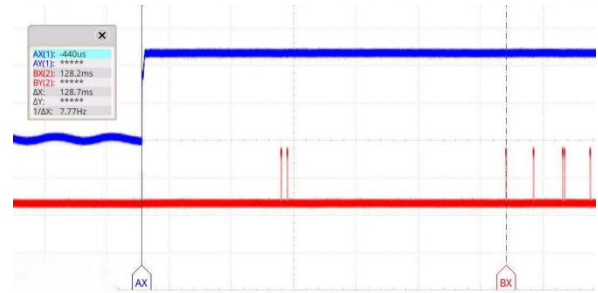
图 5-6. 样品 6 启动时间测试曲线
