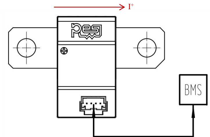
图 9-3. 低压端推荐使用场景
