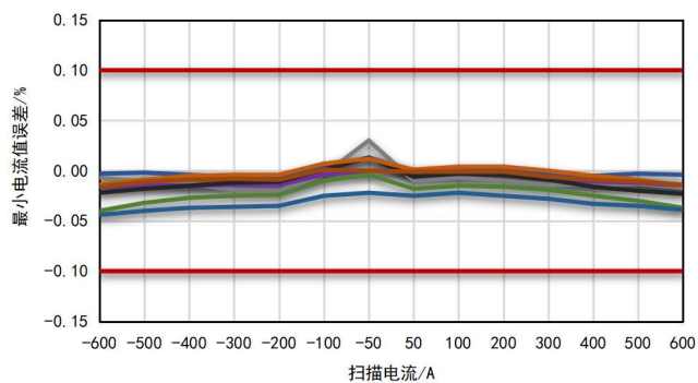
图 5-23. 85°C大电流测试精度@最小电流值误差
