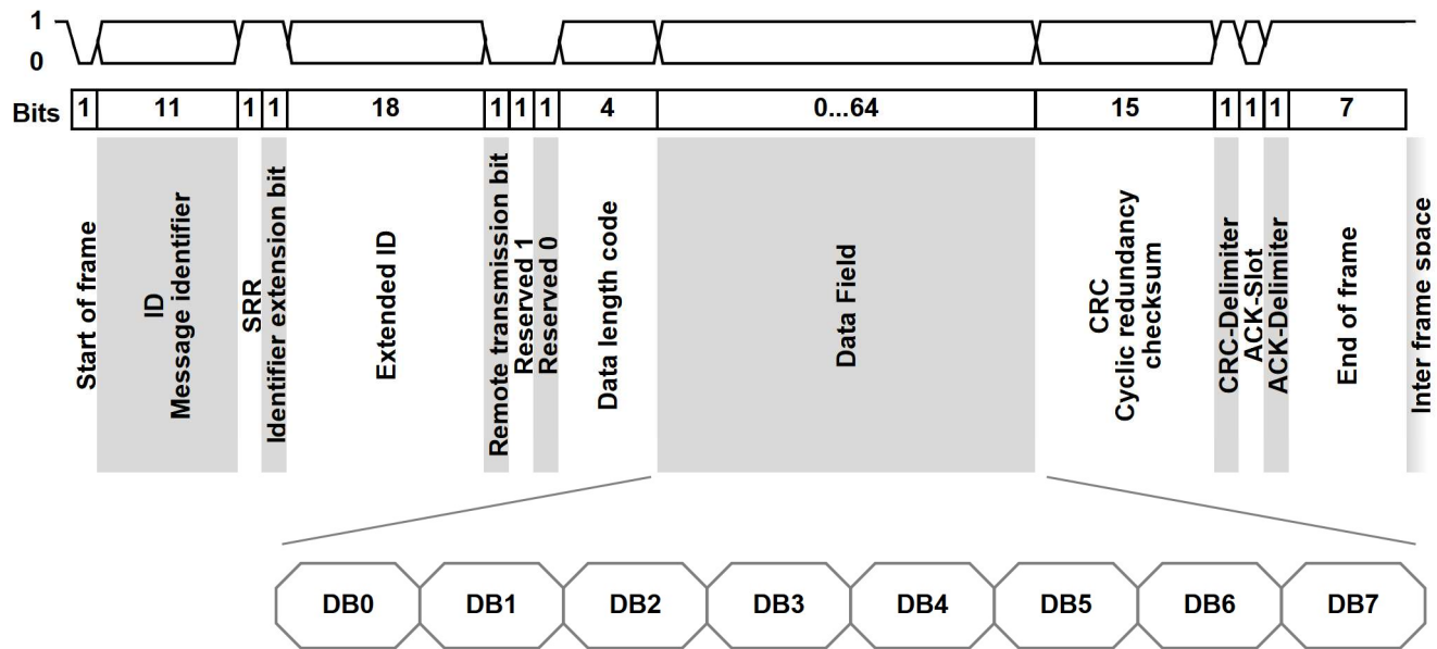
图 7-2. 扩展帧
