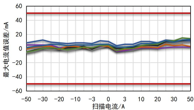
图 5-18. 105°C小电流测试精度@最大电流值误差
