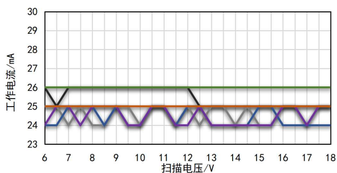
图 5-9. 25°C工作电流曲线
