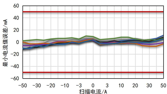
图 5-13. -40°C小电流测试精度@最小电流值误差
