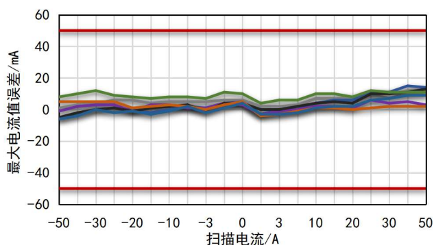
图 5-14. -40°C小电流测试精度@最大电流值误差
