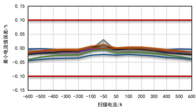
图 5-21. 25°C大电流测试精度@最小电流值误差
