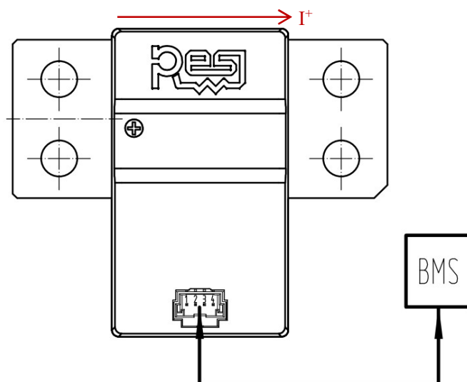
图 9-3. 低压端推荐使用场景
