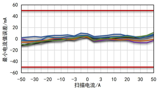
图 5-17. 105°C小电流测试精度@最小电流值误差
