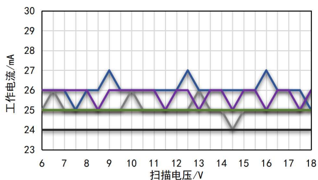
图 5-10. -40°C工作电流曲线
