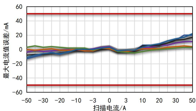
图 5-16. 25°C小电流测试精度@最大电流值误差
