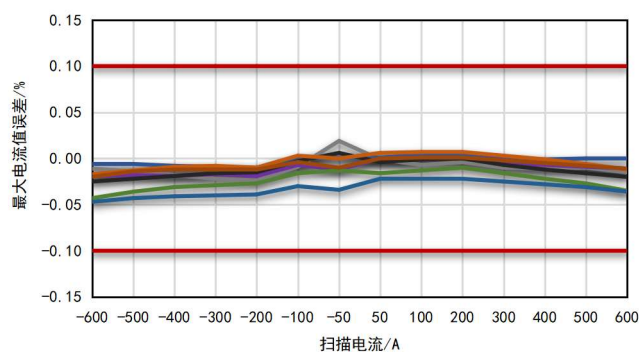
图 5-22. 25°C大电流测试精度@最大电流值误差
