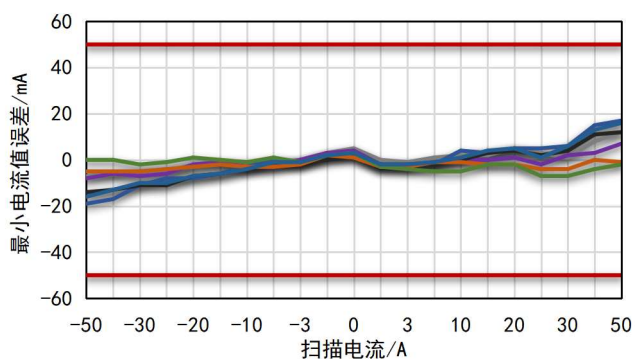
图 5-15. 25°C小电流测试精度@最小电流值误差
