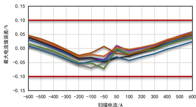
图 5-20. -40°C大电流测试精度@最大电流值误差
