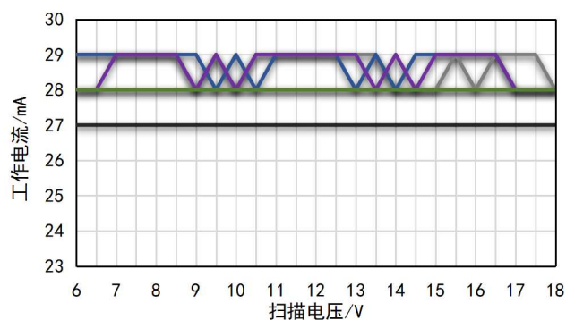
图 5-11. 105°C工作电流曲线
