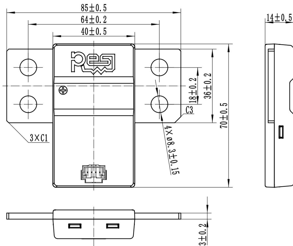
图 8-1. 结构示意图
