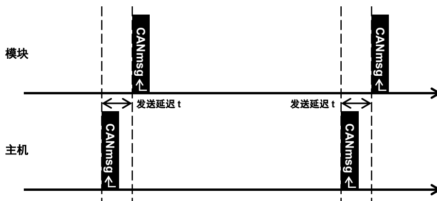
图 7-5. 命令触发模式
