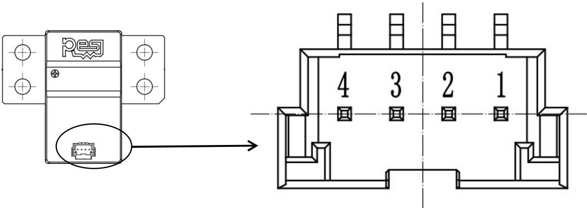
图 8-5. 公头连接器 Molex5600200420
