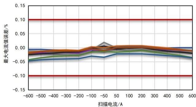
图 5-24. 85°C大电流测试精度@最大电流值误差
