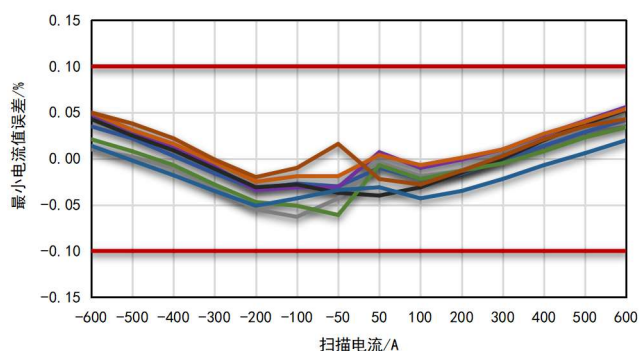
图 5-19. -40°C大电流测试精度@最小电流值误差
