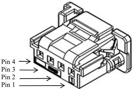
图 8-4. 母头连接器（线束端参考）
