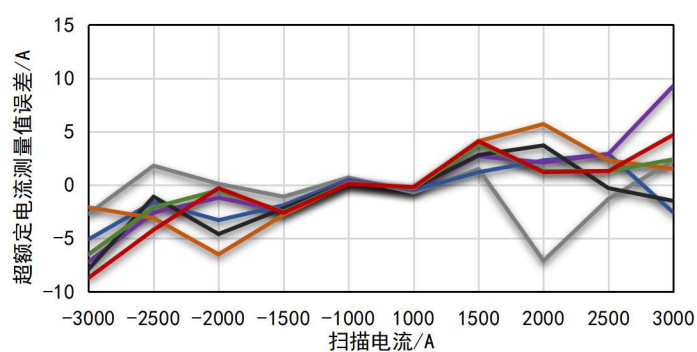
图 5-12. 25°C超额定电流测试曲线
