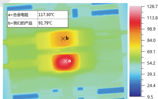
1206尺寸CSER系列箔技术电阻和同尺寸合金电阻加载1W功率后的发热对比
