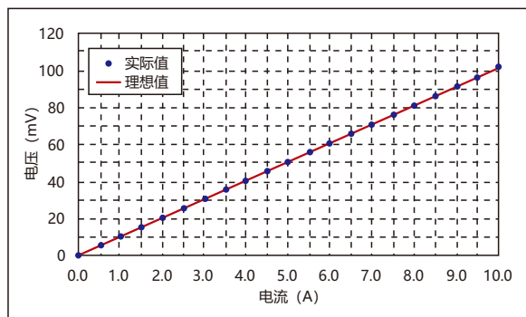
CSKR1206 尺寸 10mΩ 样品
