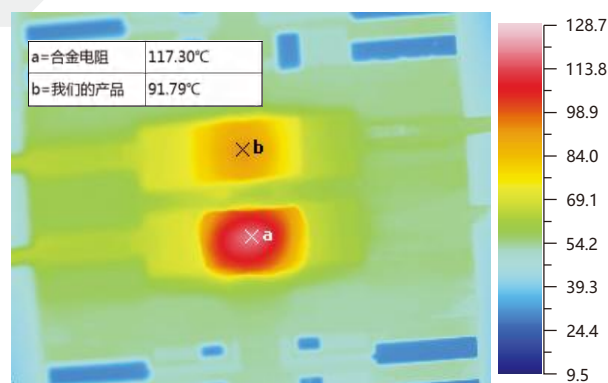
1206尺寸CSKR系列箔技术电阻和同尺寸合金电阻加载1W功率后的发热对比
