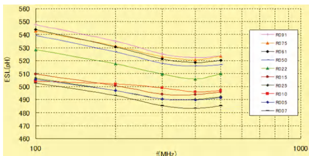
CSKR 系列串联电感参数 (单位: pH)
