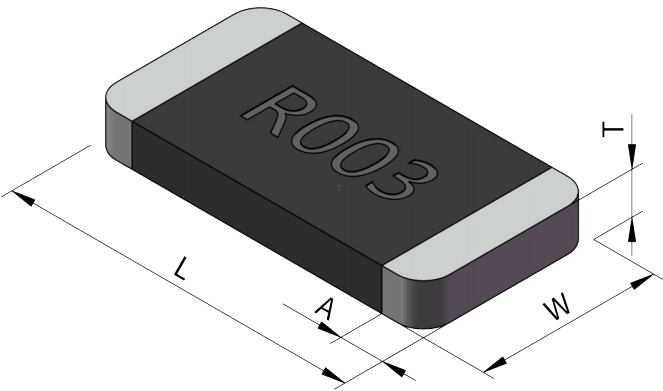
3mΩ~4mΩ标准图尺寸
