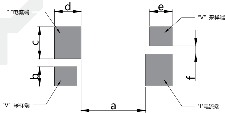
推荐焊盘尺寸
