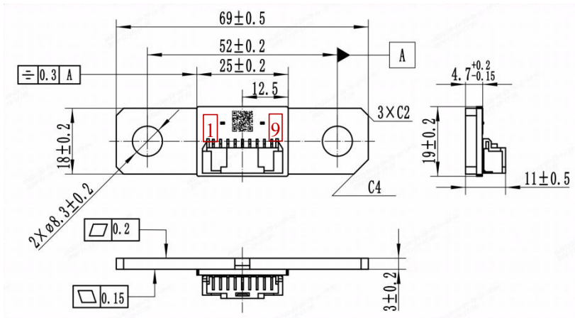
图 8-1. PCBS6918A050T2AC00 电流检测模块结构示意图
