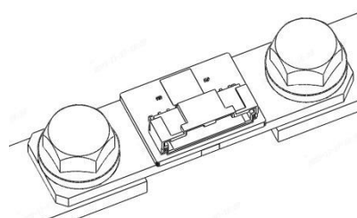
图 8-2. 铜排连接示意图
