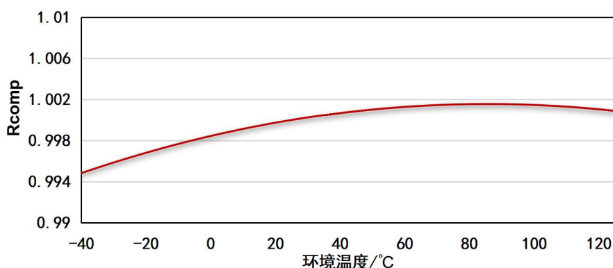
图 7-1. R COMP 温度特性曲线
