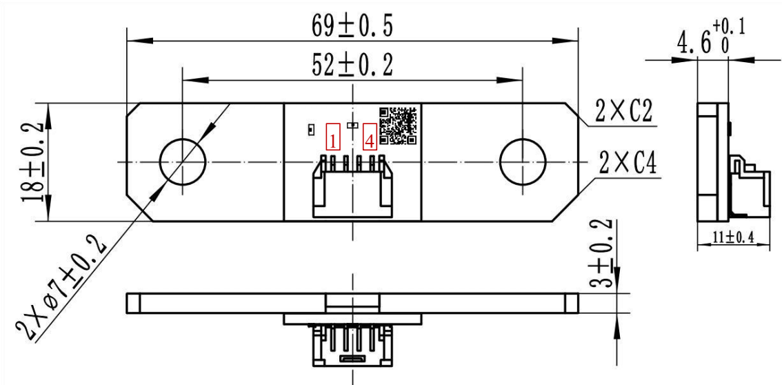
图 8-1. PCBS6918B100P2AC00 电流检测模块结构示意图
