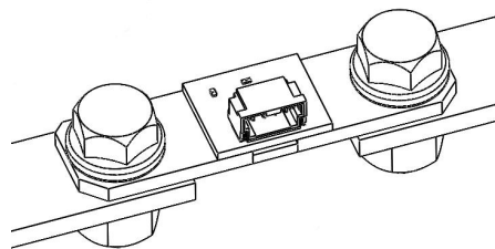
图 8-2. 连接示意图
