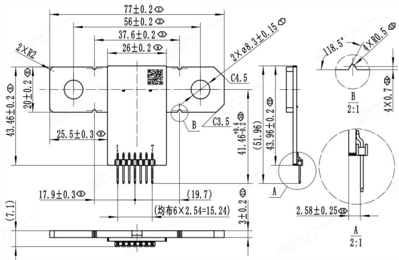
图 8-1. 结构示意图
