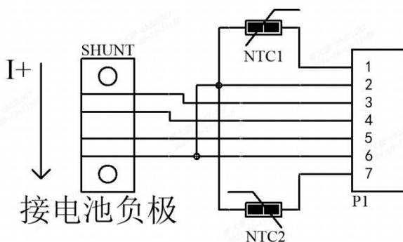
图 8-2. PCB 板原理示意图
