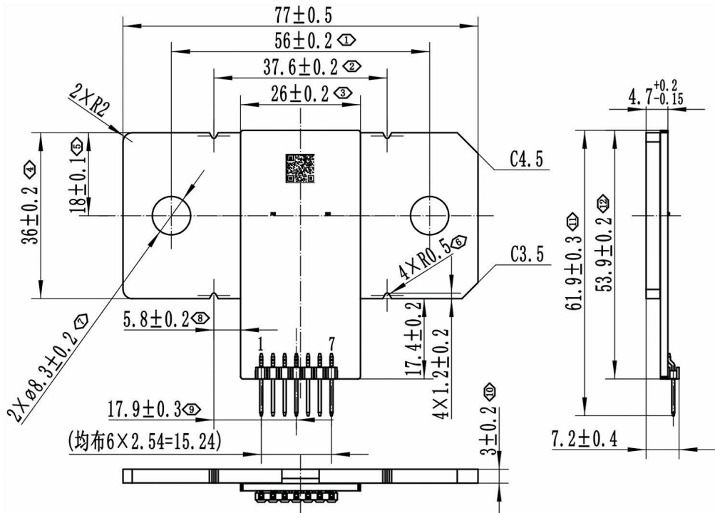
图 8-1. 结构示意图
