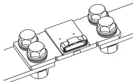
图 8-2 8436 分流器连接示意图
