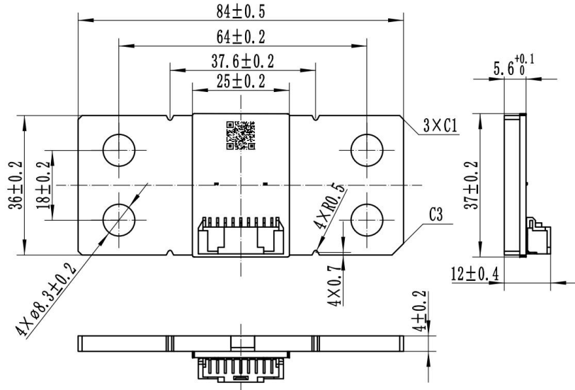
图 8-1. PCBS8436P025T0SC00 电流检测模块结构示意图
