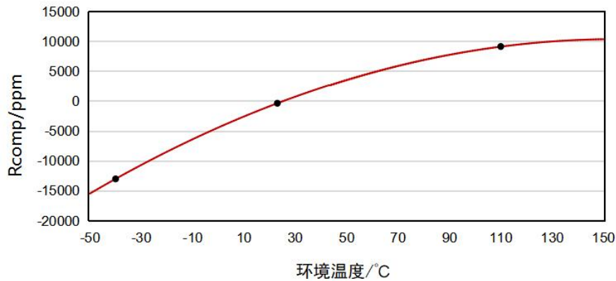
图 7-1. R COMP 温度特性曲线
