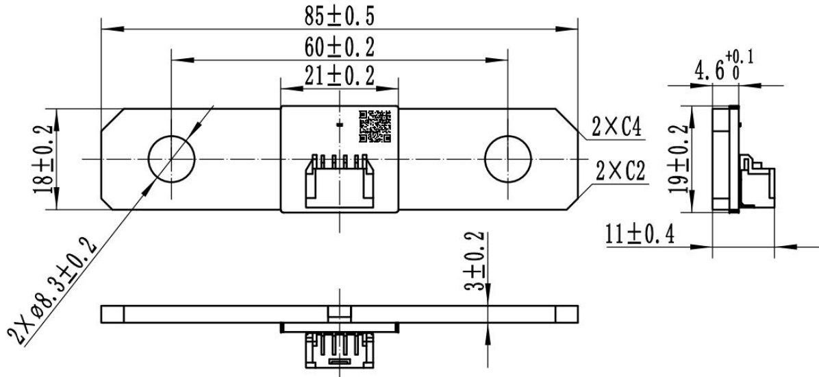
图 8-1. PCBS8518A050P1SC00 电流检测模块结构示意图
