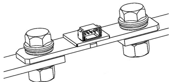
图 8-2 8518 分流器连接示意图
