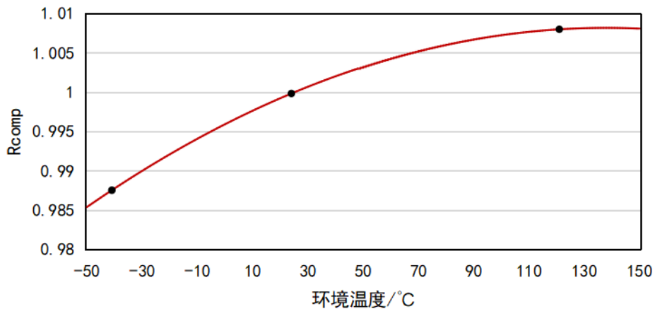
图 7-1. R_{COMP} 温度特性曲线
