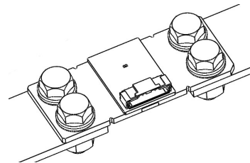
图 8-2 8536 分流器连接示意图
