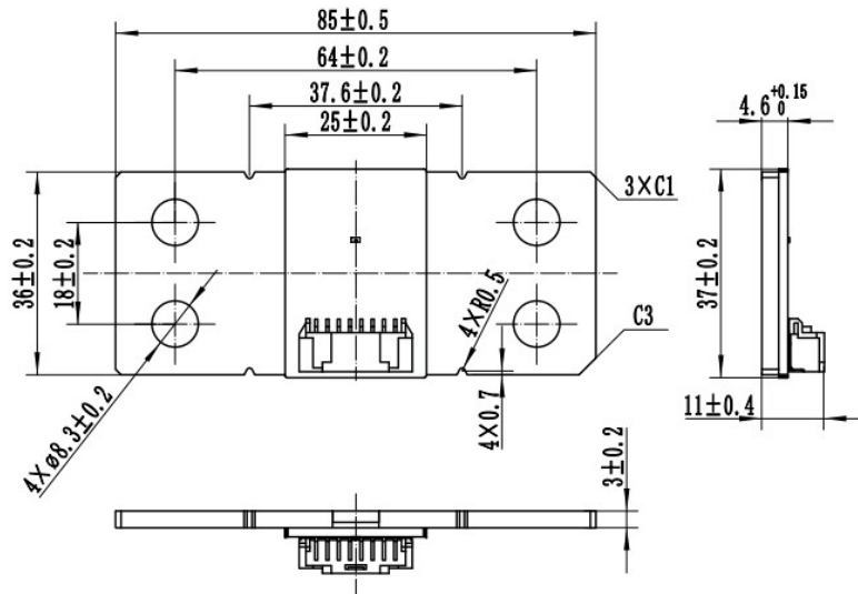
图 8-1. PCBS8536P050S1SC00 电流检测模块结构示意图
