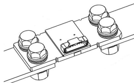
图 8-2 8536 分流器连接示意图
