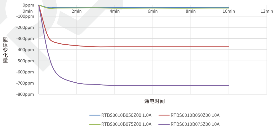
RTBS0010系列分流器通电电阻值变化情况
