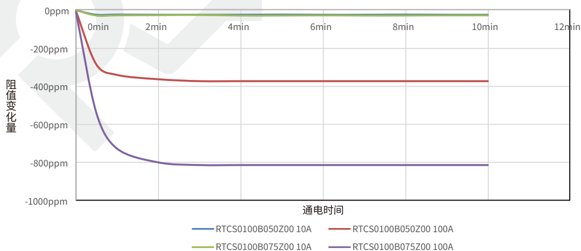
RTCS0100系列分流器通电电阻值变化情况
