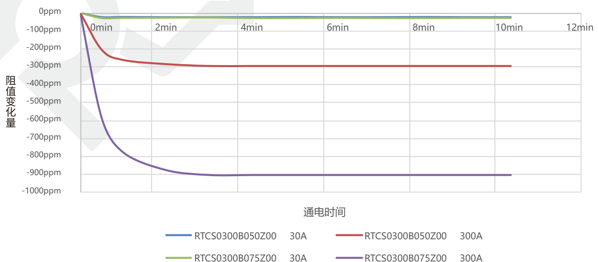
RTCS0300系列分流器通电阻值变化情况
