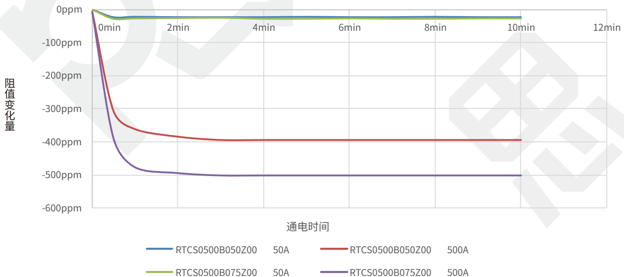
RTCS0500系列分流器通电电阻值变化情况
